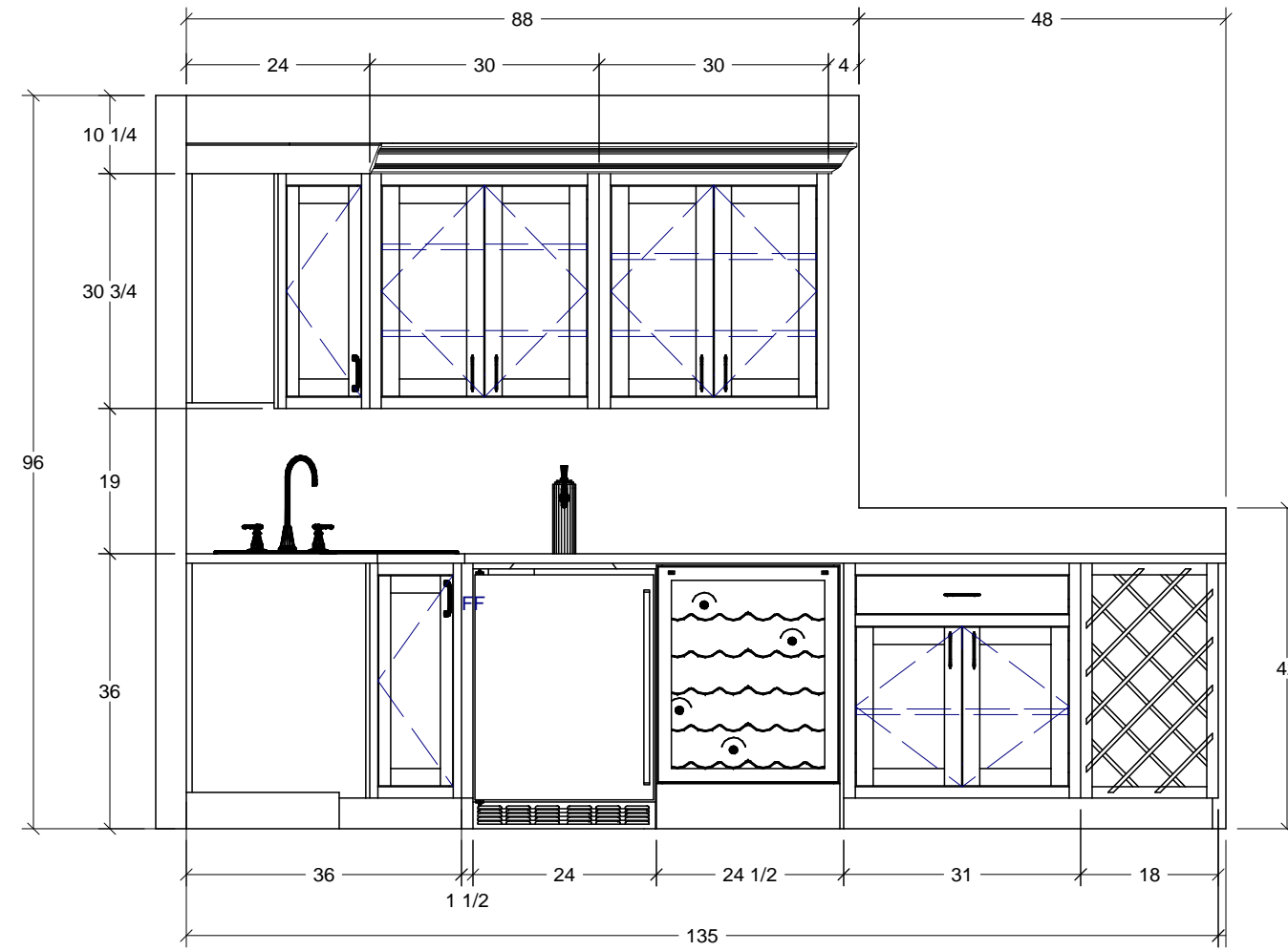
2 Elevation Wall 2 Scale: 1/2" = 1'
