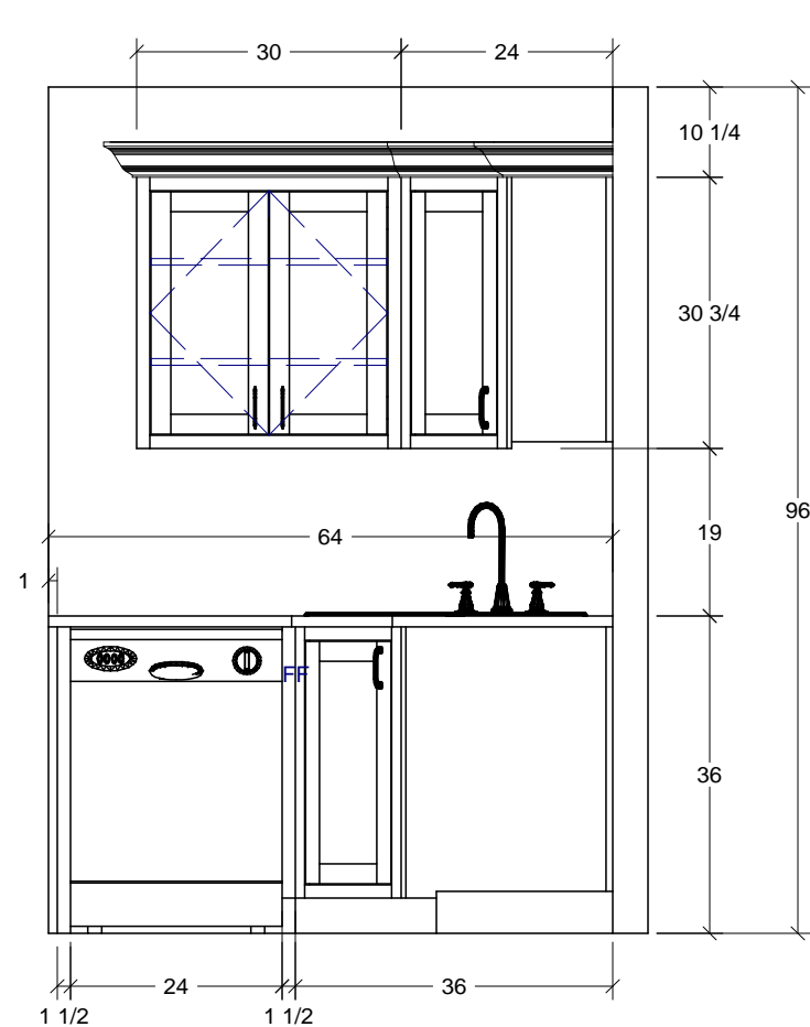
1 Elevation Wall 1 Scale: 1/2" = 1'
